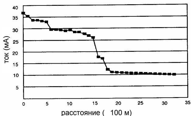
Изменение потерь тока по длине линии
